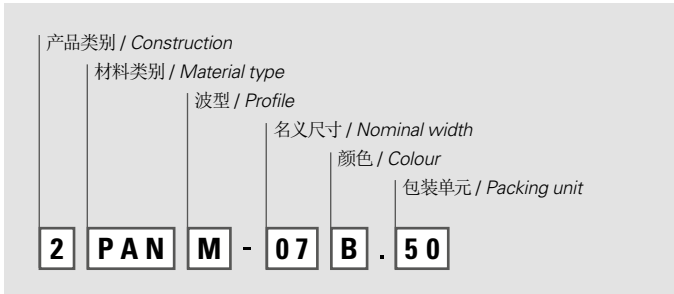
中间波型 M / Intermediate profile M
