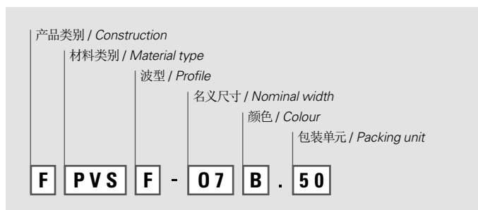
细波型 F / Fine profile F
